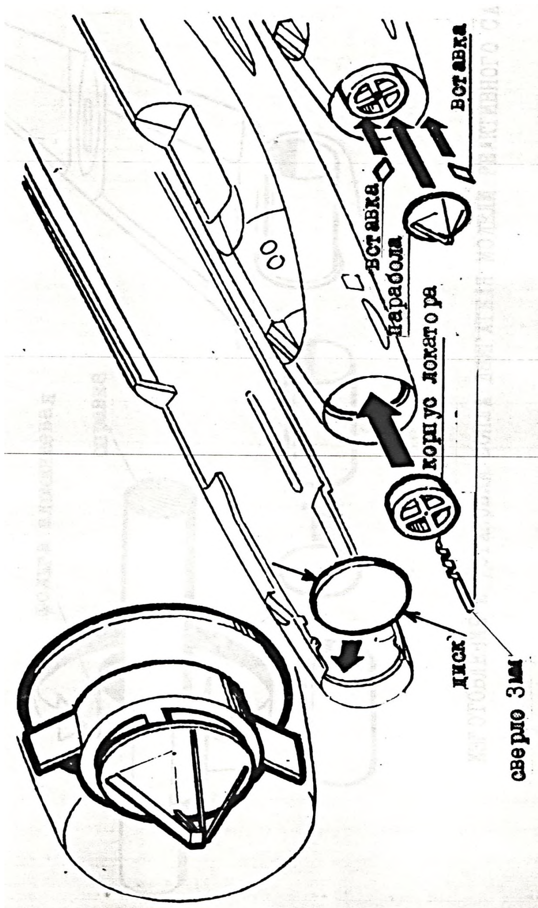
Изготовление и установка входного устройства на модель реактивного самолёта
