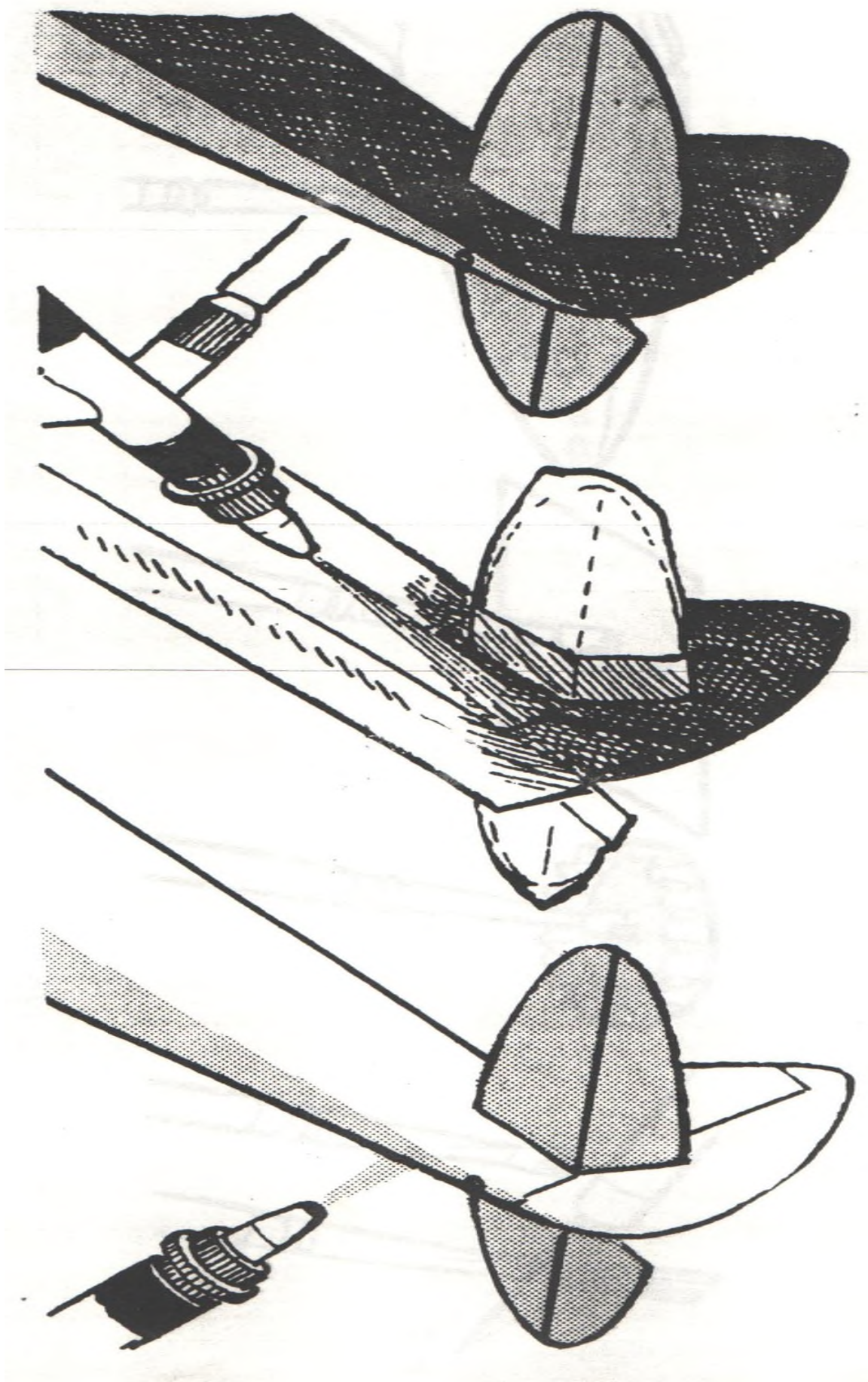
Разделение окрашиваемых поверхностей с помощью липкой ленты
