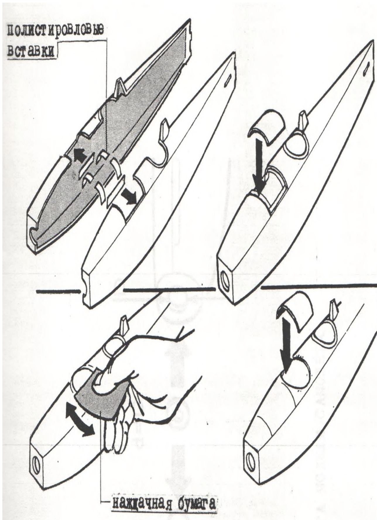
Переделка двухместного самолёта в одноместный
